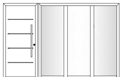
Cotim 11 Fixe en dormant 3 vitrages.
